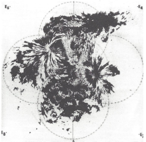
Die Bewegung der drei äußeren Planeten The Movement of the Three Superior Planets
